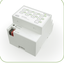
CELLIO KNX Product Code: K.CEL.01Z.20N.WO 8-fold binary input - dry contacts / Ingresso Binario 8 Canali - contatto pulito
